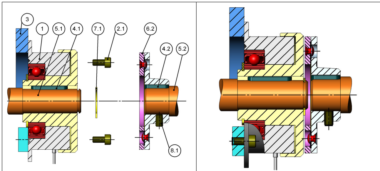
Abbildung 5: Wellenmontierte Kupplung mit Flansch & Ankerteil Nabenhals außen (z. B. 06...07-03-230-xxxx)
