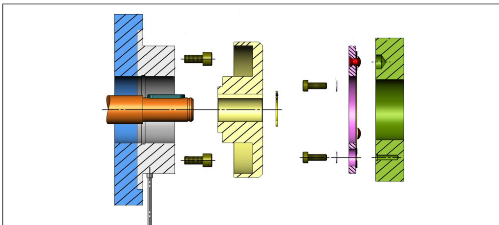
Abbildung 15: Kupplung demontieren (Beispiel Ausführung 110)
