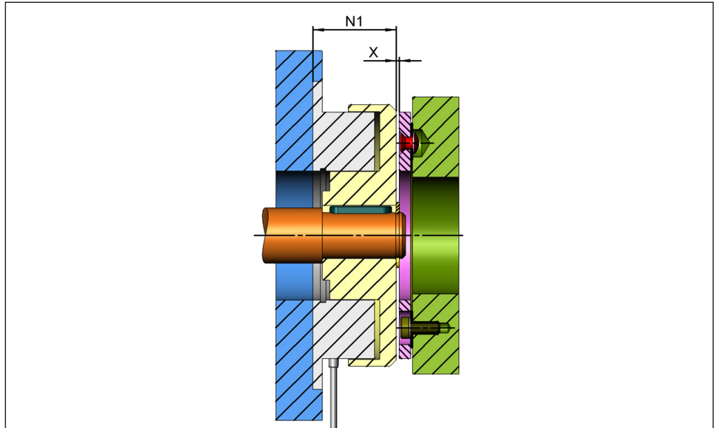
Abbildung 16: Kontrolle des Luftspaltes
