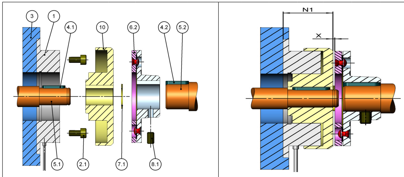
Abbildung 3: Flanschmontierte Kupplung mit Ankerteil - Nabenhals außen (z. B. 01...12-03-130-xxxx)
