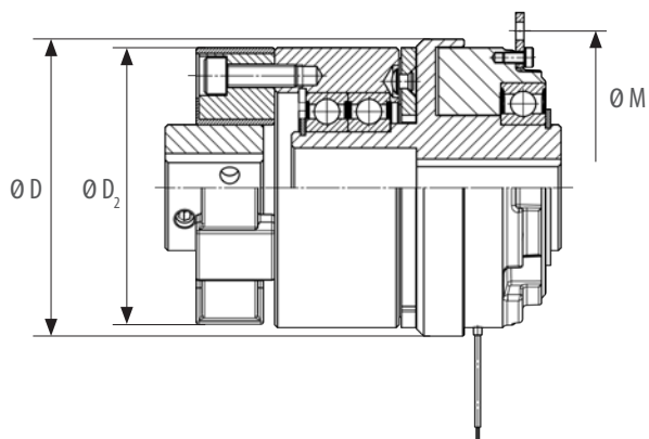
Wellenmontiert (Baugröße 08-12)
