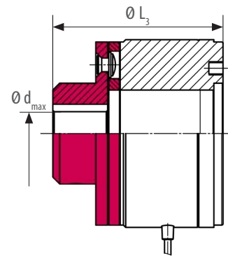
Nabenhs außen (Ausführung 30)
