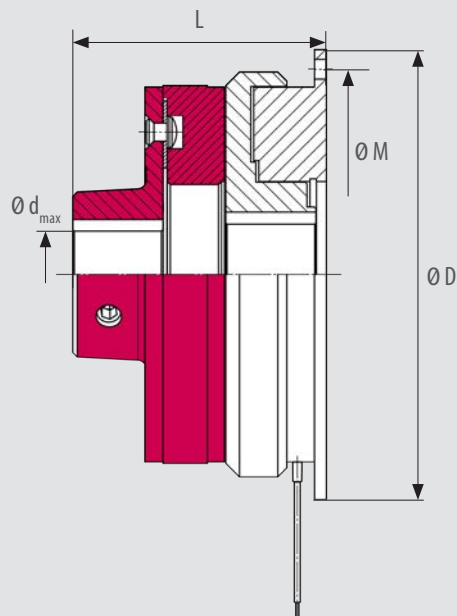
Nabenhals außen (Variante 130)
