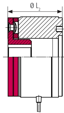
Nabenhs im Magneten (Ausführung 20)
