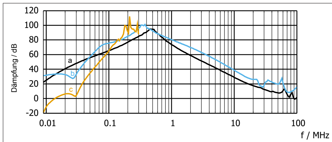
Abb. 4: 20E6T60-30xx Einfügungsdämpfung
