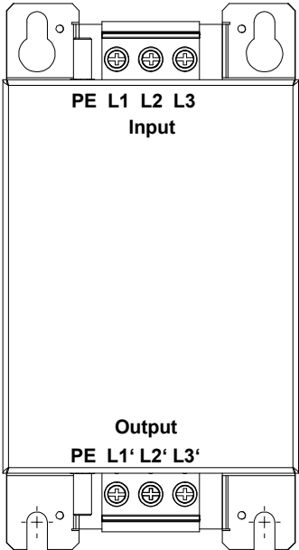
Abb. 9: Anschluss 18...20E6T60-30xx
