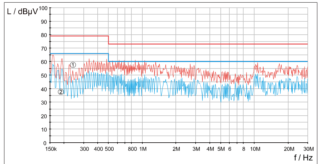
Abb. 13: 20E6T60-30xx Störspannungsmessung C2 4kHz 100m
