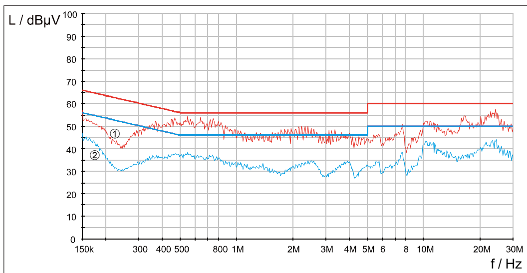
Abb. 12: 20E6T60-30xx Störspannungsmessung C1 4kHz 50m
