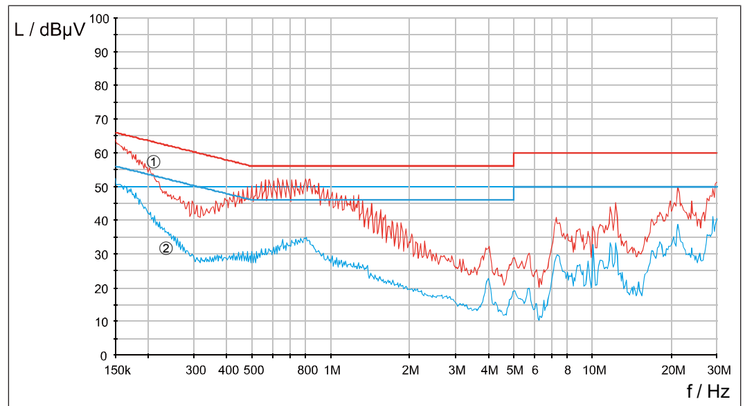
Abb. 10: 18E6T60-30xx Störspannungsmessung C1 4kHz 50m
