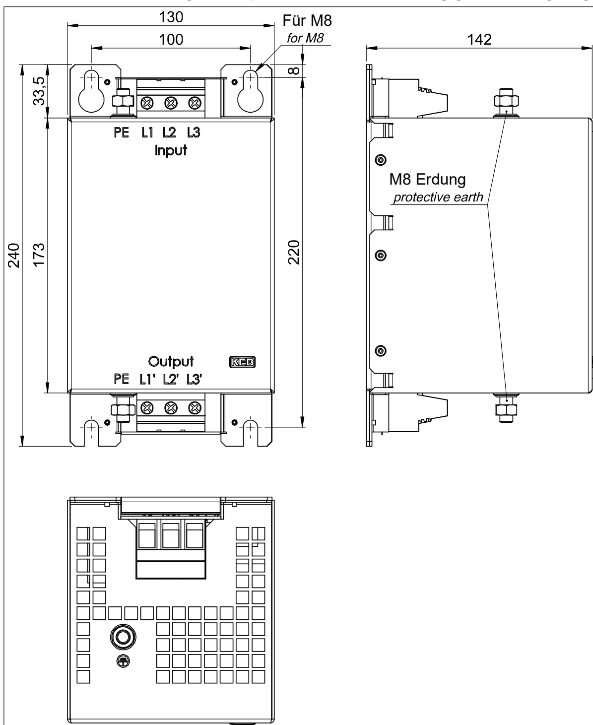
Abb. 6: Abmessungen 18E6T60-30xx
