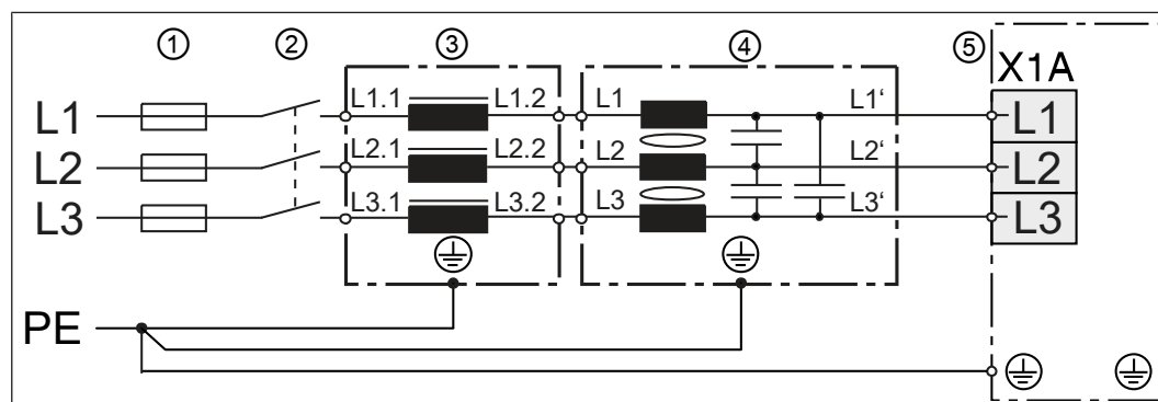
Abb. 8: Anschluss 3ph Drossel-Filter-FU
