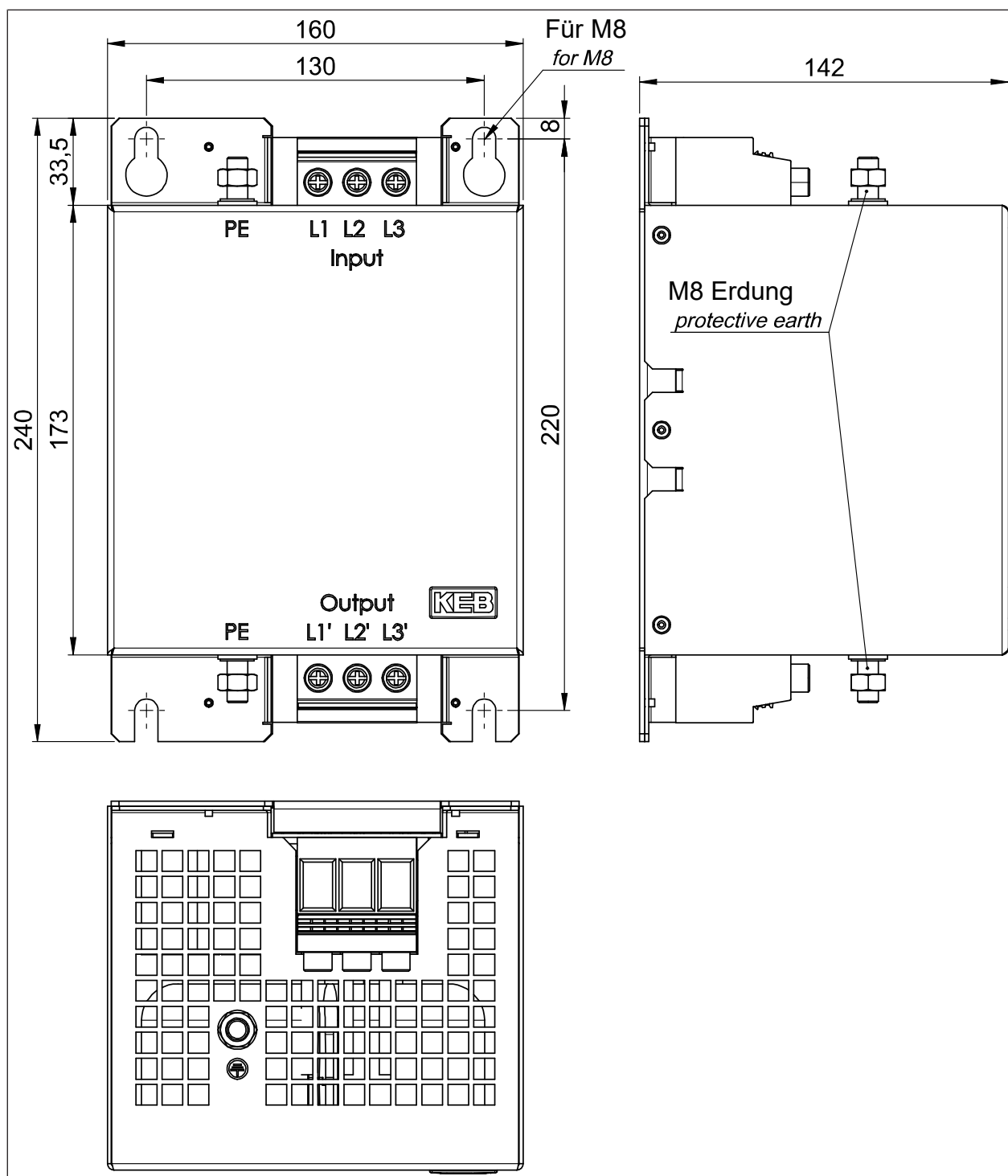
Abb. 7: Abmessungen 20E6T60-30xx
