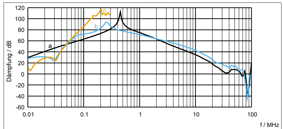
Abb. 3: 18E6T60-30xx Einfügungsdämpfung
