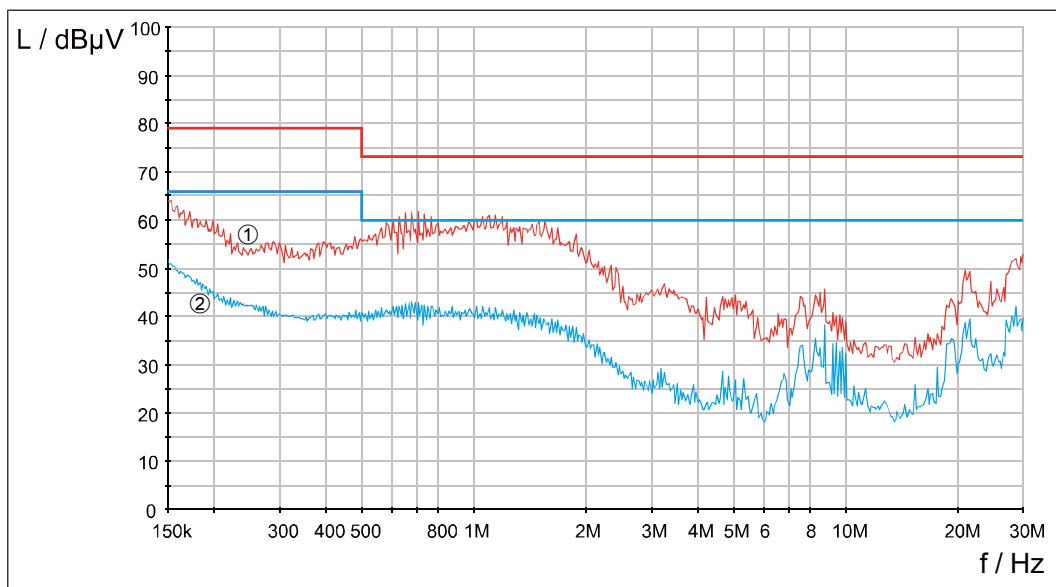
Abb. 11: 18E6T60-30xx Störspannungsmessung C2 4kHz 100m
