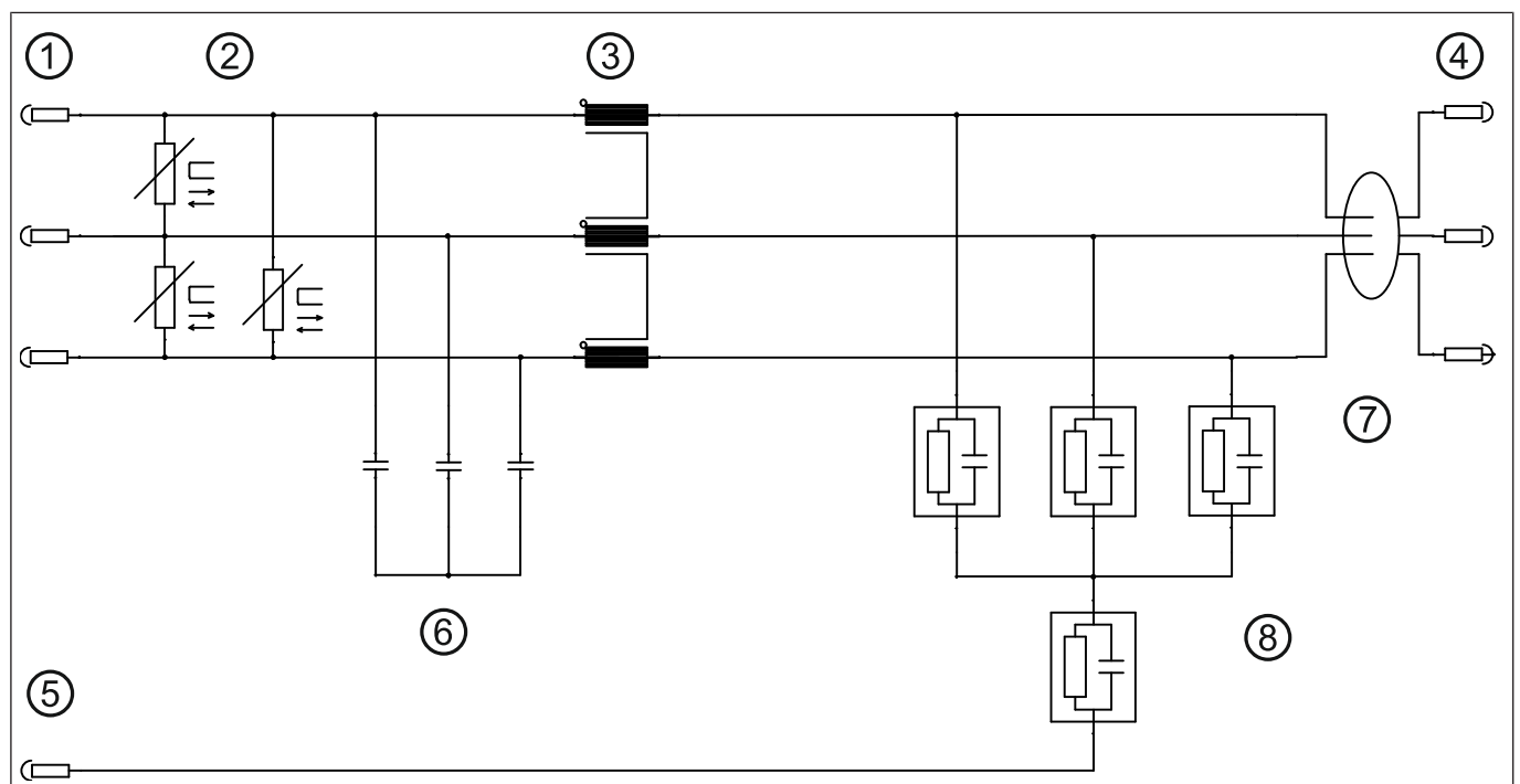
Abb. 1: Prinzipschaltbild TN/TT-Netz
