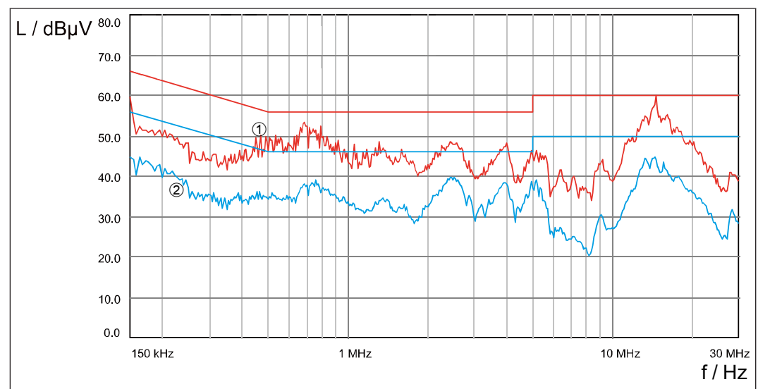
Abb. 8: 24E6T60-30xx Störspannungsmessung C1 4kHz 50m
