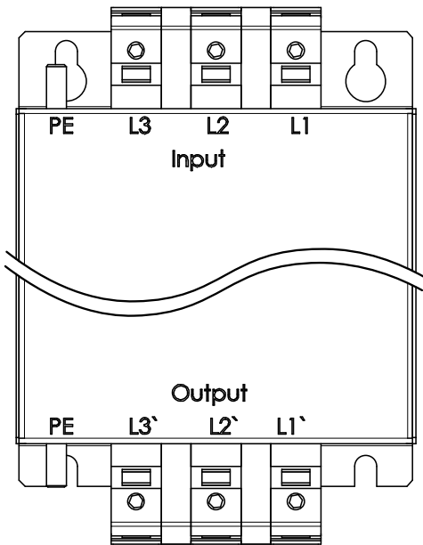
Abb. 5: Anschluss 22...24E6T60-30xx
