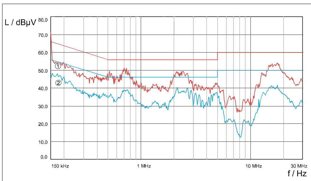
Abb. 6: 22E6T60-30xx Störspannungsmessung C1 4kHz 50m
