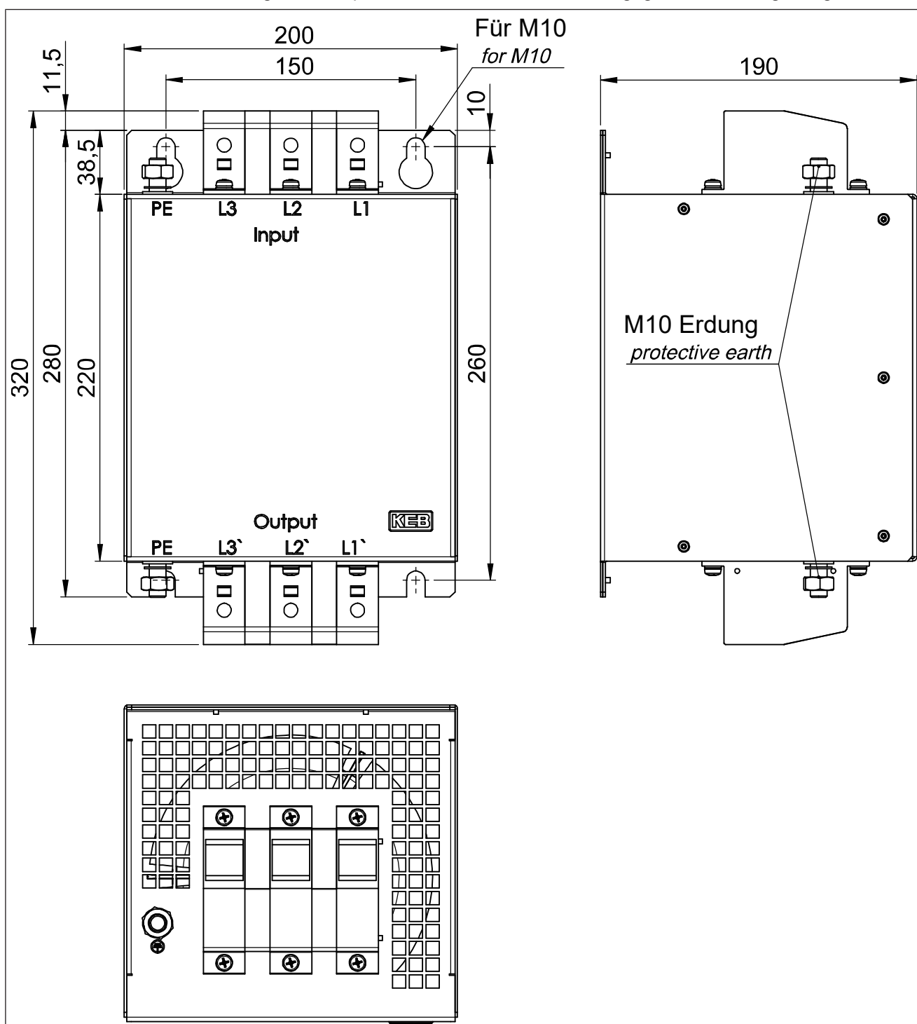
Abb. 3: Abmessungen 22...24E6T60-3000
