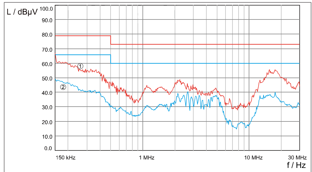
Abb. 7: 22E6T60-30xx Störspannungsmessung C2 4kHz 100m
