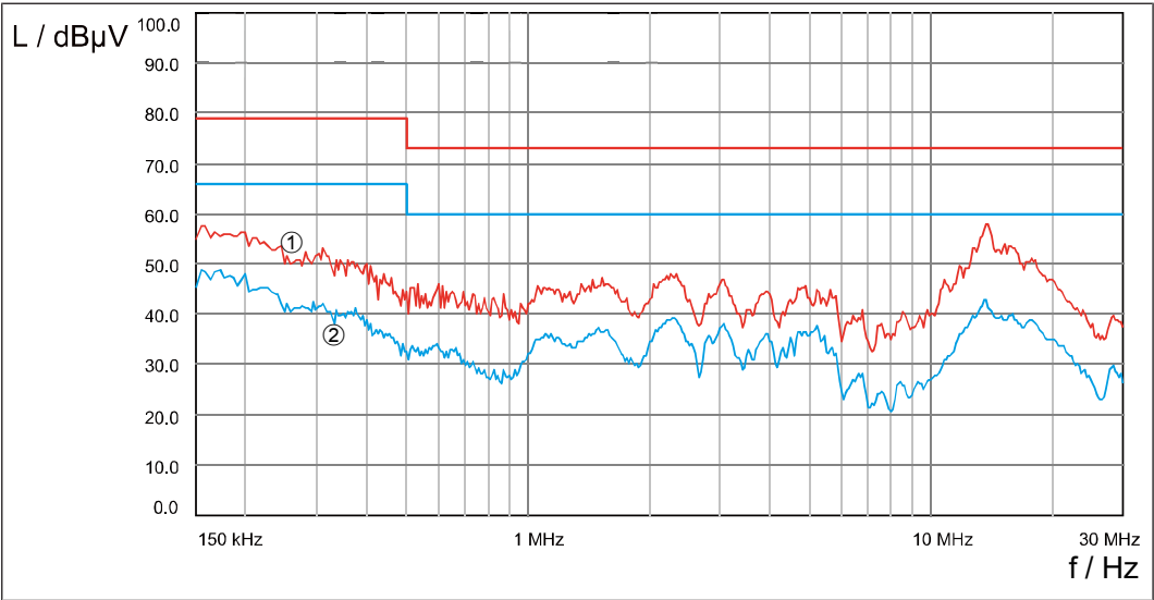
Abb. 9: 24E6T60-30xx Störspannungsmessung C2 4kHz 100m
