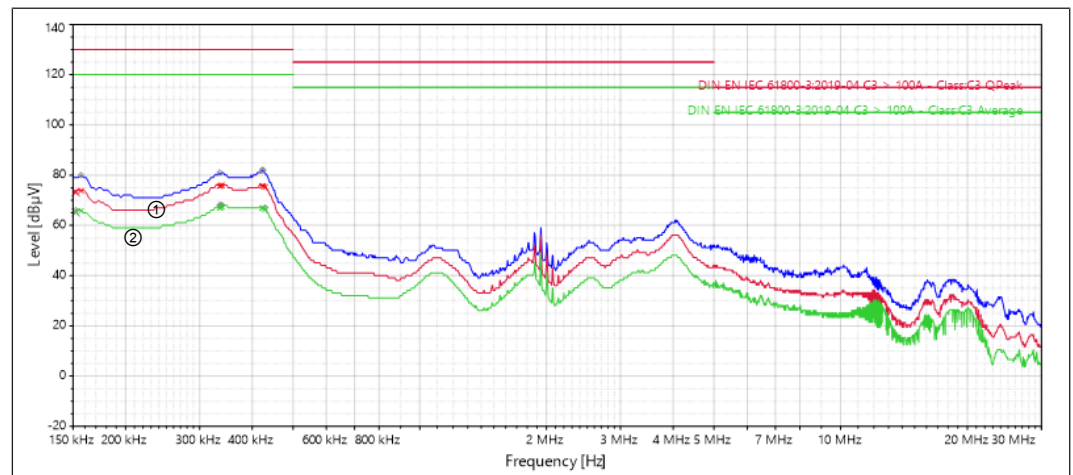
Abb. 8: 33E6T60-3150 Störspannungsmessung C3 4kHz 100m
