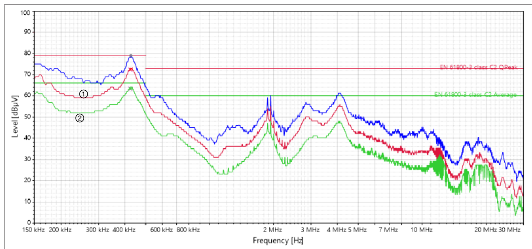
Abb. 7: 33E6T60-3150 Störspannungsmessung C2 4kHz 50m
