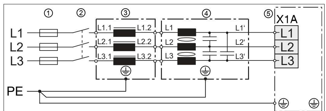
Abb. 5: Anschluss 3ph Drossel-Filter-FU
