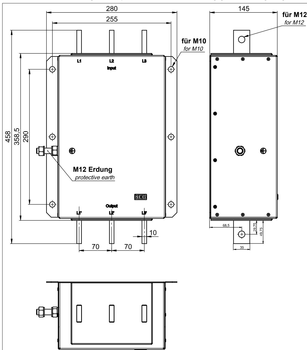
Abb. 4: Abmessungen 33E6T60-3150
