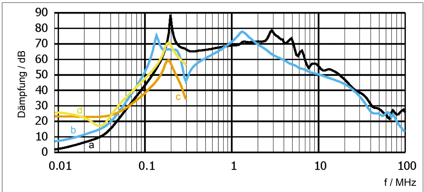
Abb. 2: 33E6T60-3150_Dämpfung
