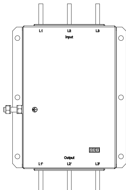
Abb. 6: Anschluss 33E6T60-3150
