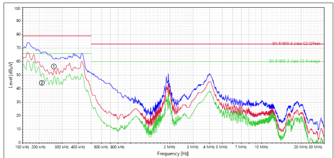
Abb. 9: 33E6T60-3150 Störspannungsmessung C2 8kHz 100m
