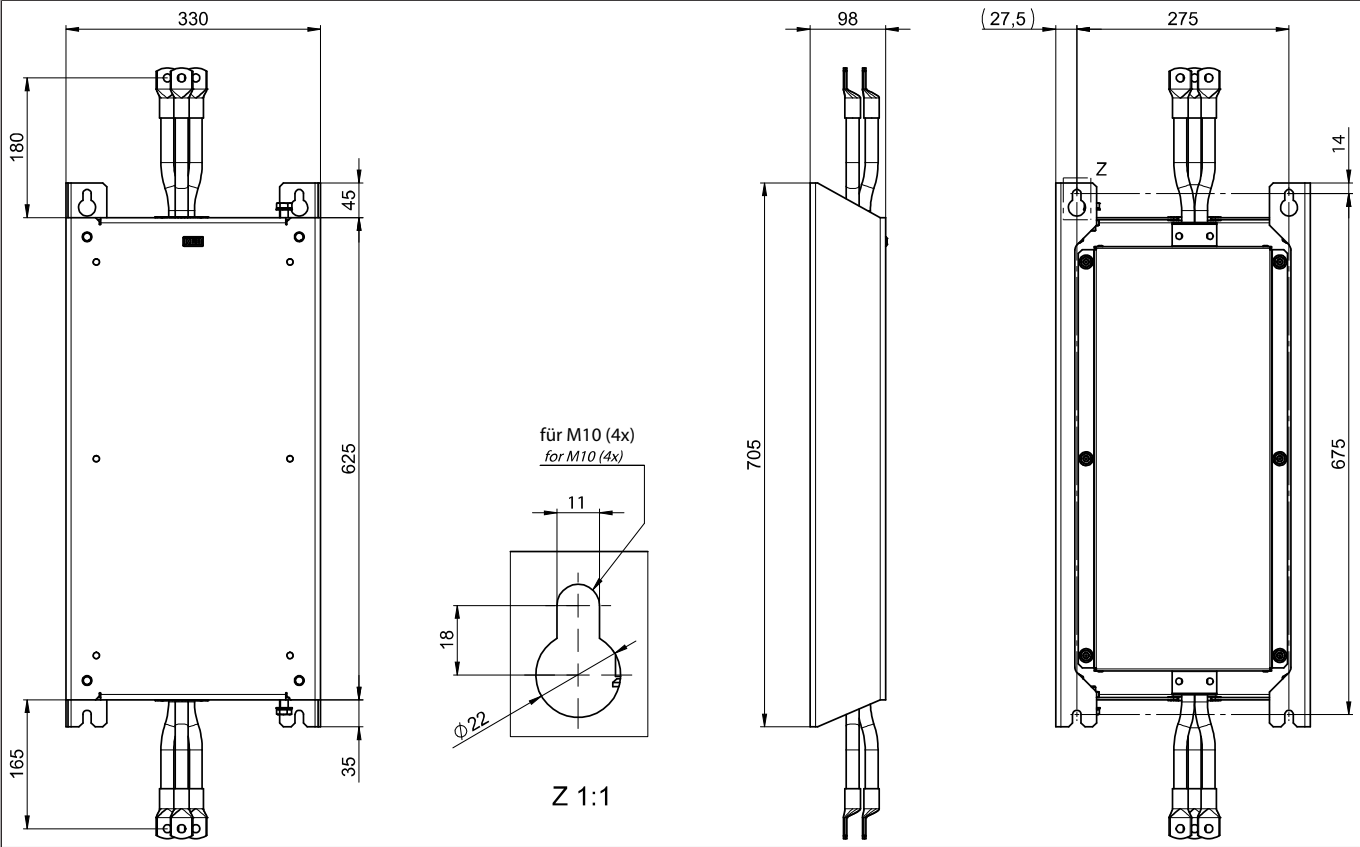
Abb. 6: Abmessungen 27E6T60-1150
