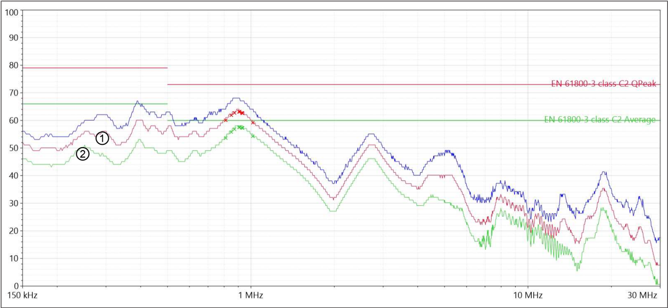
Abb. 9: 27E6T60-1150 Störspannungsmessung C2
