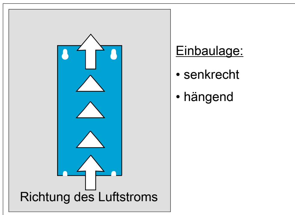
Abb. 3: Zulässige Einbaulage
