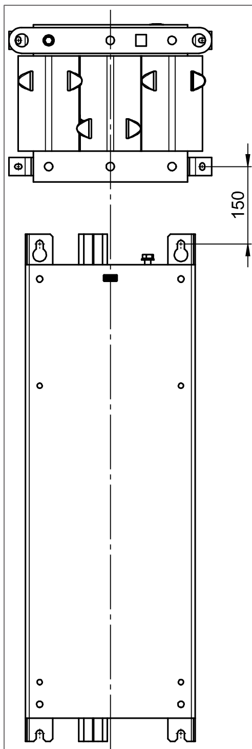
Abb. 5: Einbauabstand zwischen HF-Filter und Netzdrossel
