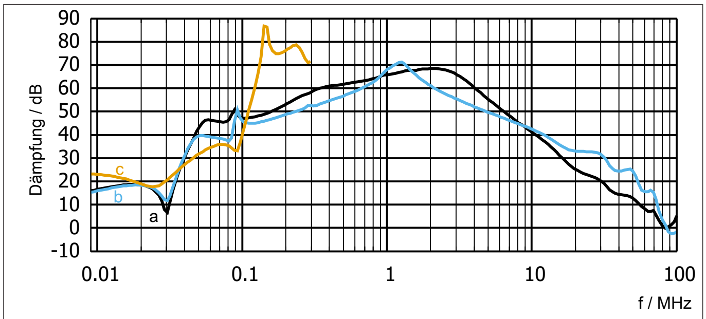
Abb. 2: Einfügungsämpfung 27E6T60-1150
