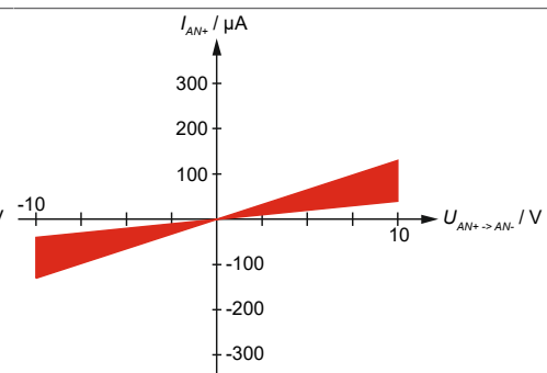
Differenzielle Spannungsmessung
