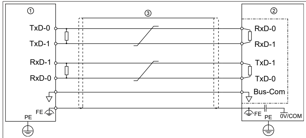
Abb. 7: Anschlussbeispiel RS485 mit internem Abschlußwiderstand 4-Wire 2 Knoten
