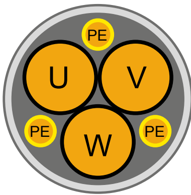
Abbildung 28: Symmetrische Motorleitung
