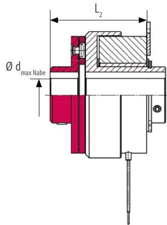
Nabenhals außen (Variante 630)
