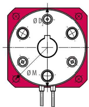
Rechteckflansch (Variante 200)
