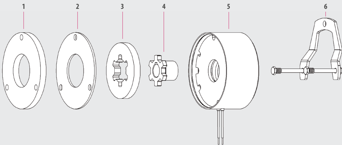
1. Flansch 2. Reibscheibe 3. Belag 4. Nabe 5. Magnetsystem 6. Handlüftung
