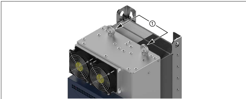
Abbildung 13: Beispiel eines F6 im Gehäuse 8 mit M10-Ringschrauben
