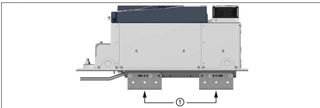
Abbildung 14: Beispiel eines F6 Gehäuse 7 mit Transportwinkeln
