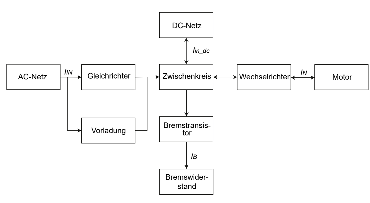
Abbildung 5: Blockschaltbild des Energieflusses
