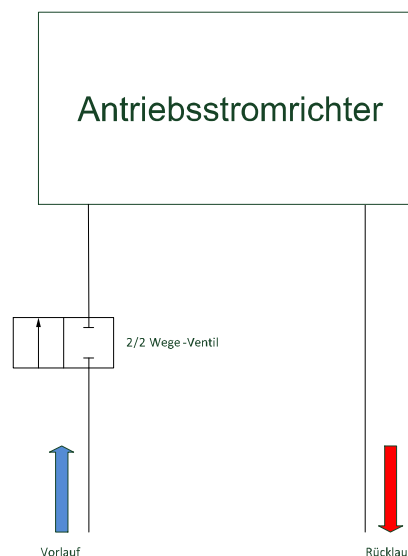
Abb. 3: Kühlmittelregelung mit 2/2-Wege-Magnetventil
