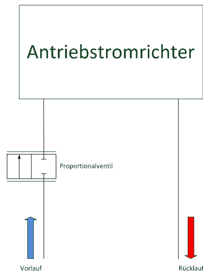
Abb. 2: Kühlmittelregelung mit 2-Wege-Proportionalventil
