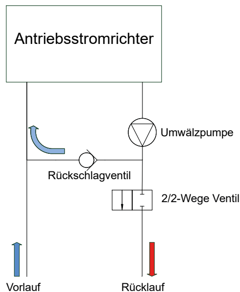
Abb. 1: Kühlmittelregelung mit Umwälzpumpe
