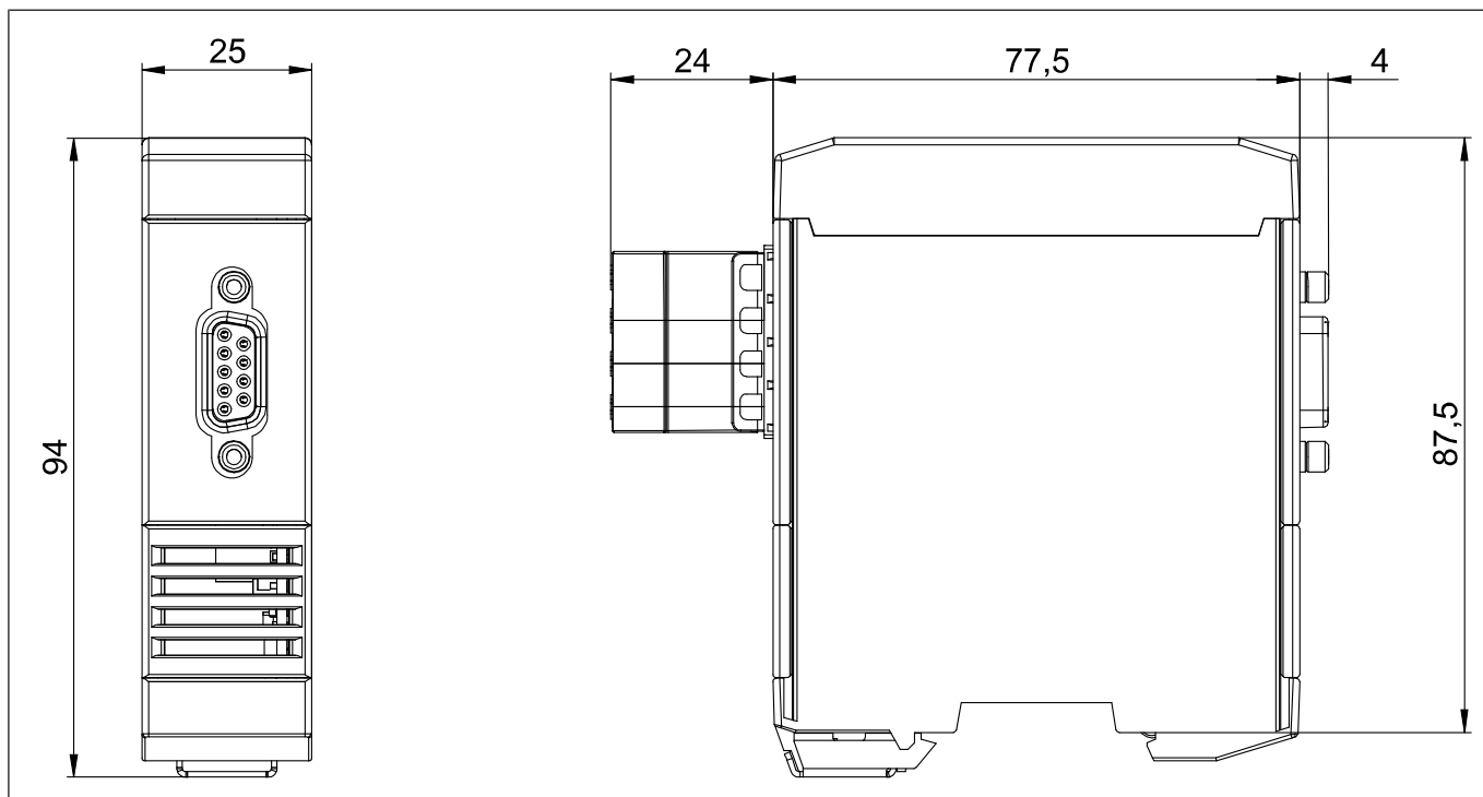
Abb. 2: Abmessungen MAINS MODULE
