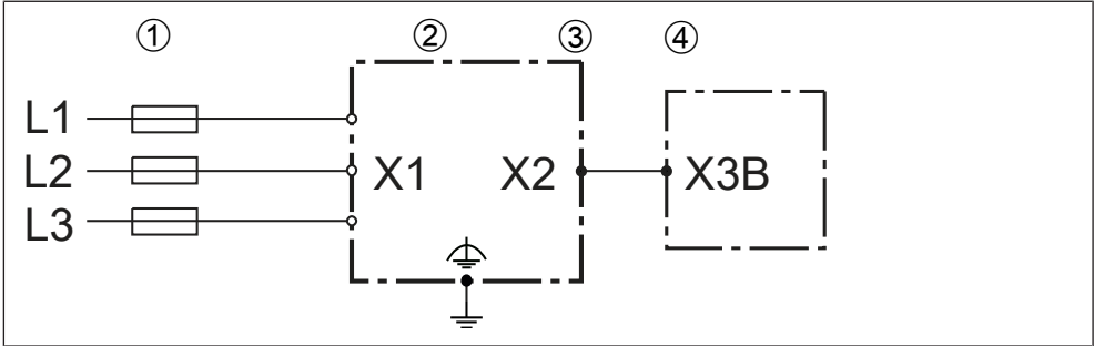
Abb. 3: Netzanschluss
