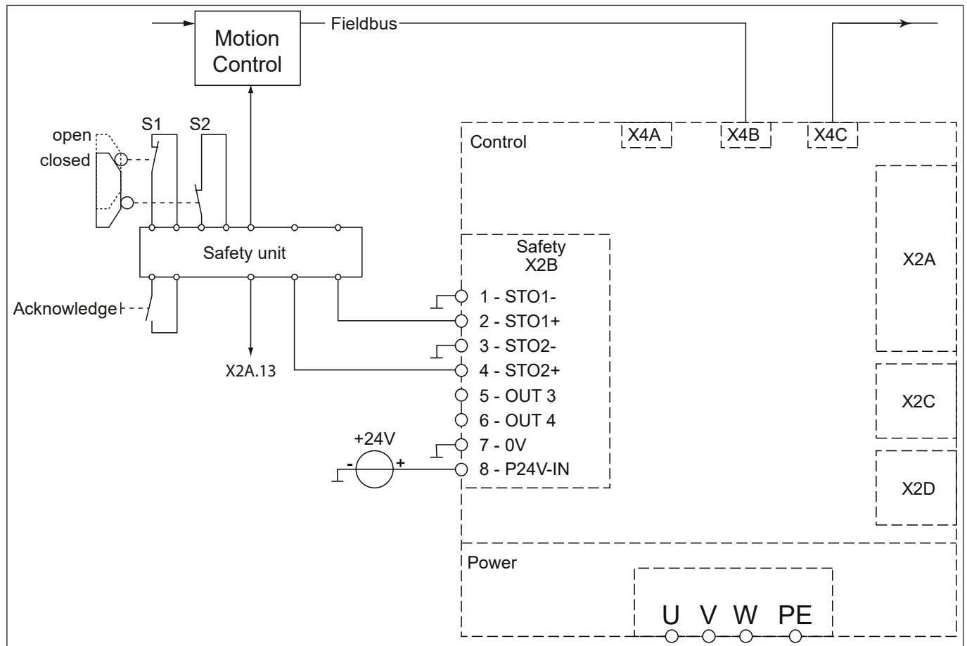
Fig. 12: Wiring_SS1
