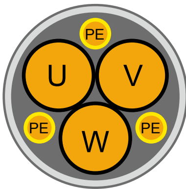
Abbildung 29: Symmetrische Motorleitung
