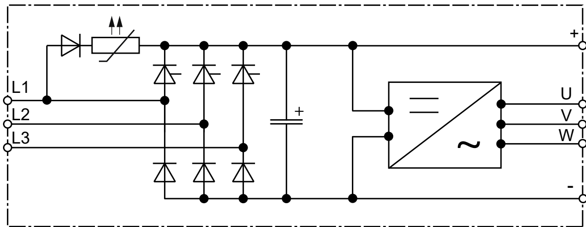
Abbildung 21: Eingangsbeschaltung
