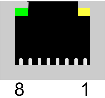
Abb. 17: Buchse RJ45 Frontansicht
