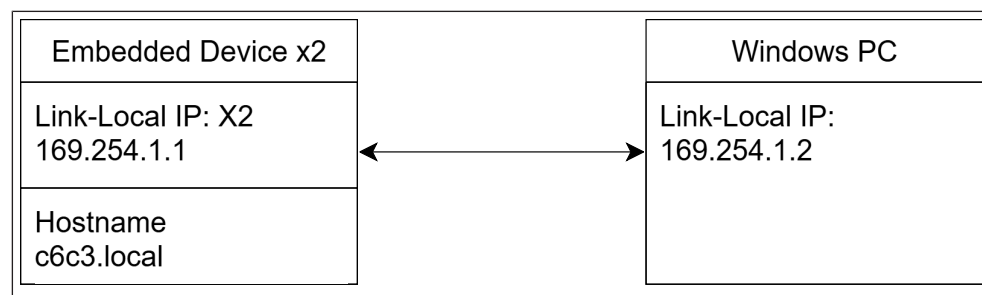
Abb. 24: P2P Verbindung
