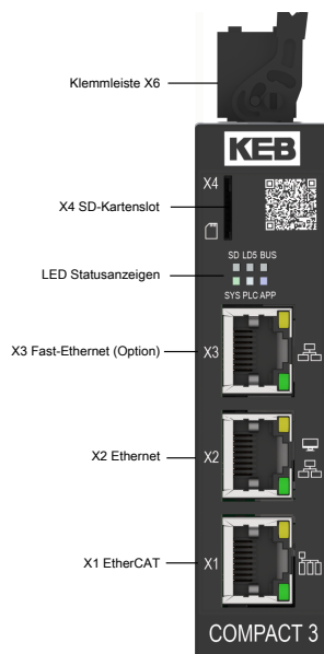
Abb. 3: C6 COMPACT 3 Frontansicht Modell 2
