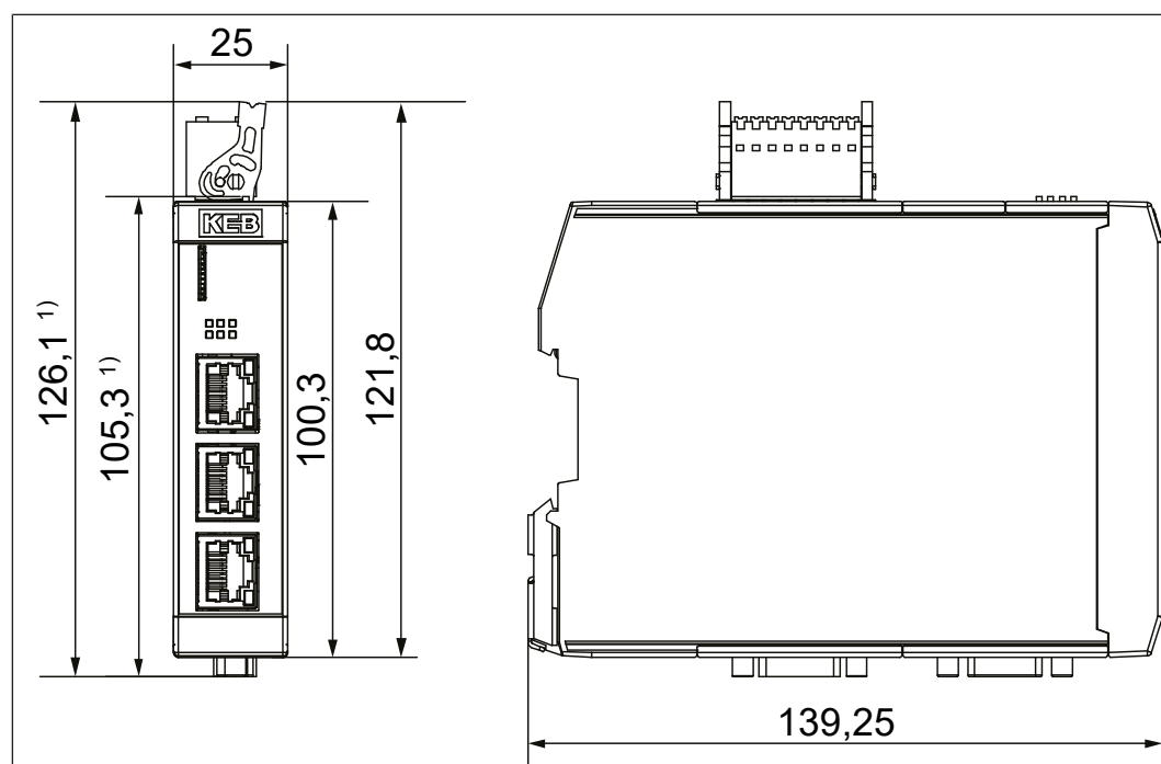
Abb. 11: Abmessungen COMPACT 3
