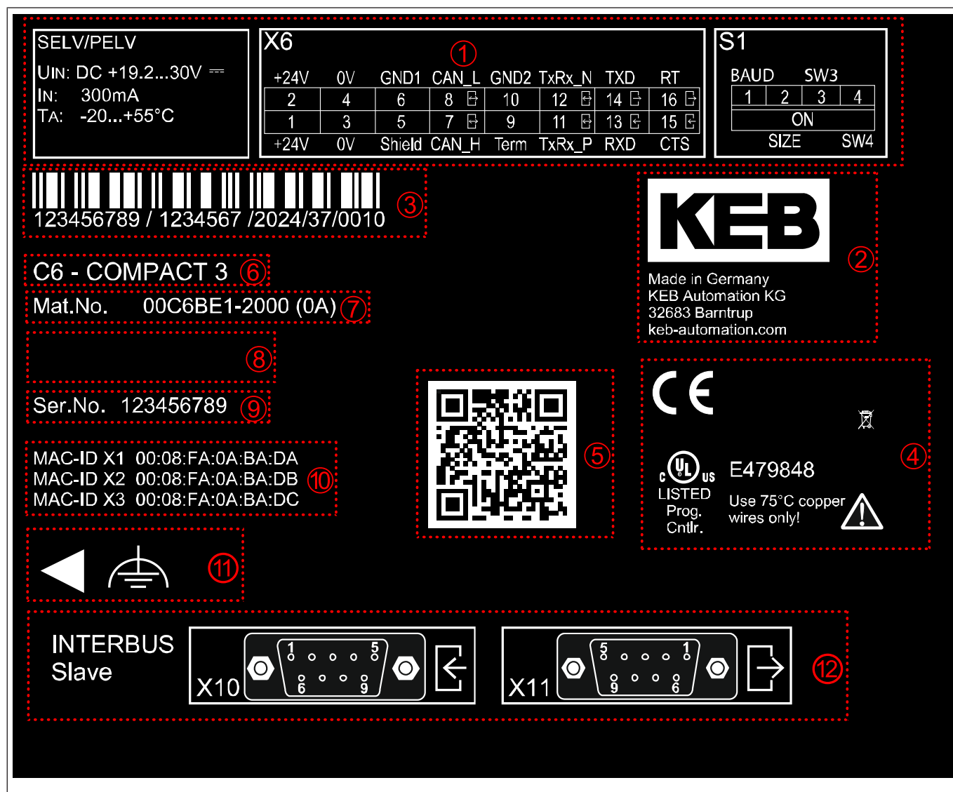
Abb. 1: Typenschild
