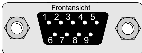
Abb. 19: X10 INTERBUS Eingang
