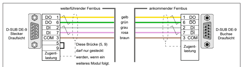
Abb. 21: Belegung INTERBUS-Fernbuskabel
