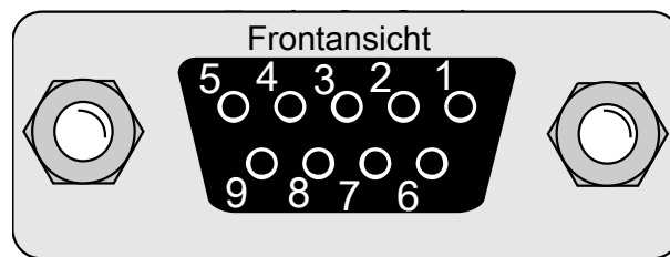
Abb. 20: X11 INTERBUS Ausgang
