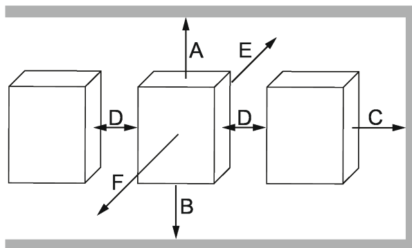
Abb. 12: Einbauabstände
