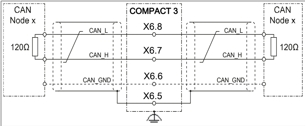
Abb. 18: Anschluss CAN-Bus
