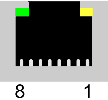
Abb. 16: Buchse RJ45 Frontansicht
