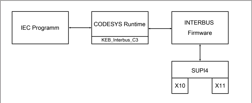
Abb. 22: Softwarestruktur INTERBUS-Erweiterung
