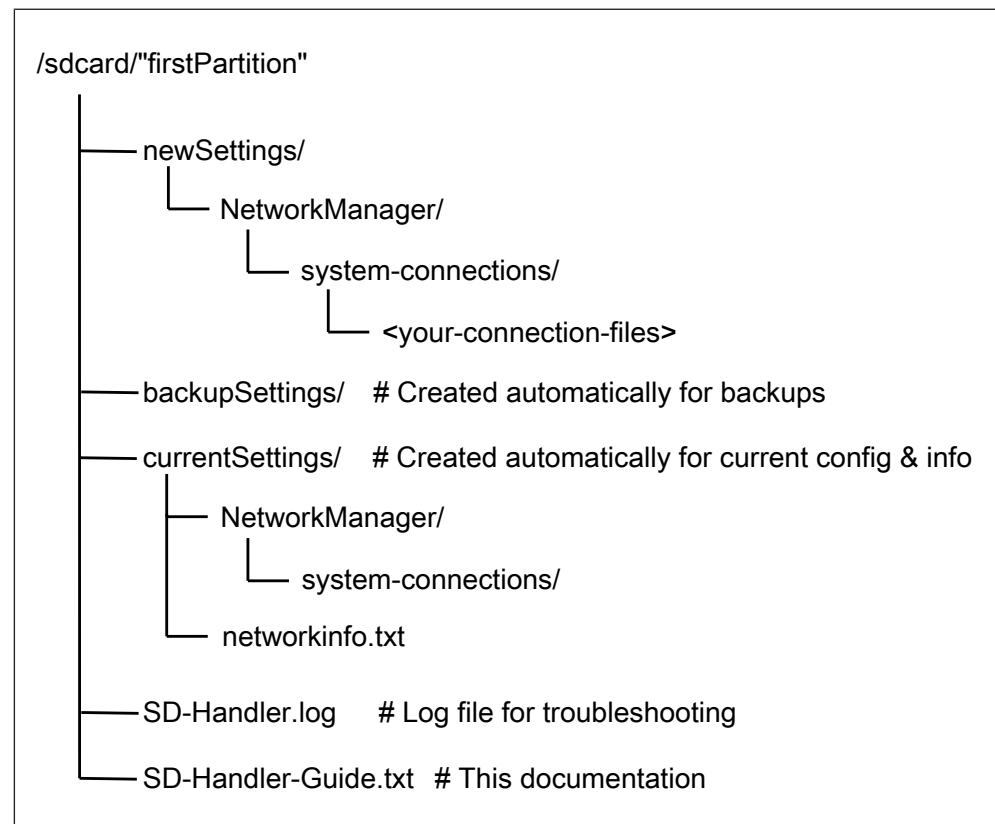
Abb. 42: Übersicht Ordnerstruktur
