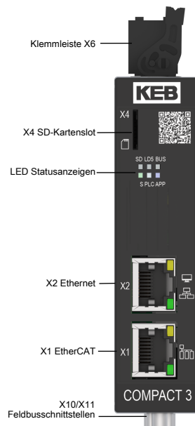
Abb. 4: C6 COMPACT 3 Frontansicht Modell 4
