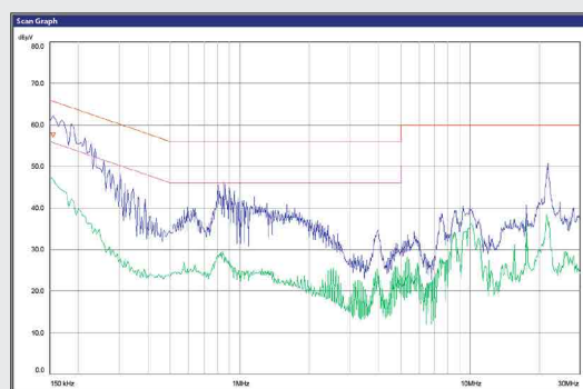
EMV-Kennlinie
