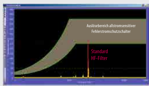
Vergleich Ableitströme
